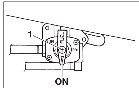
1. Винт
